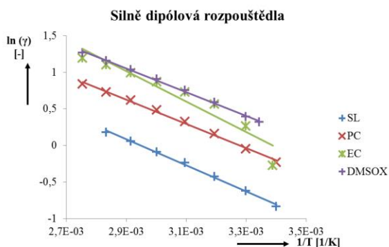
Obr.4: Graf závislosti přirozeného logaritmu měrné vodivosti silně dipólových rozpouštědel na teplotě
