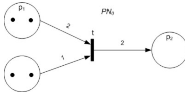
Obrázek 4.3: Petriho síť před odpálením, převzato z [Wikipedia(2015b)].
