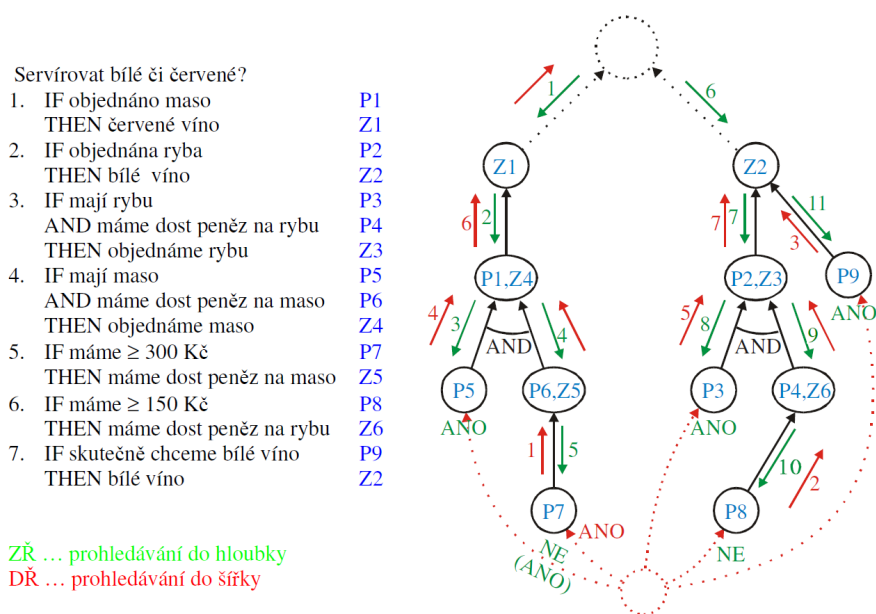
Obrázek 5.1: Příklad inferenční sítě a možnosti prohledávání, převzato z [MÜLLER(2002)].
