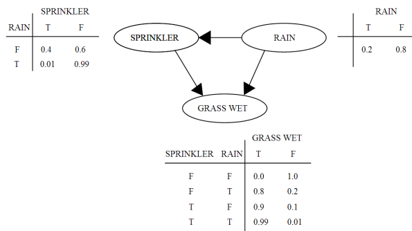
Obrázek 6.1: Příklad Bayesovské sítě, převzato z [Wikipedia(2015a)].
