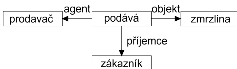
Obrázek 4.2: Příklad sémantické sítě, převzato z [LUKASOVÁ()].
