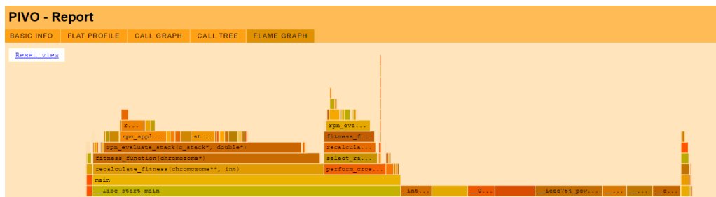
Obrázek 7.7: Flame graph generovaný nástrojem PIVO
