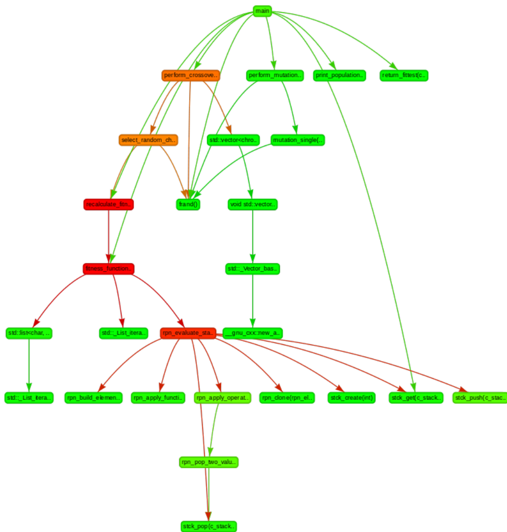
Obrázek 9.4: Call-graph zpracovaný nástrojem PIVO z běhu genetického algoritmu, uzly jsou obarveny podle inkuzivního času
