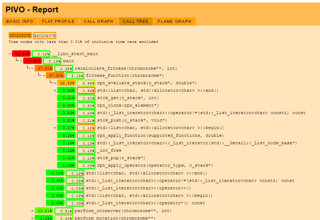
Obrázek 7.6: Call tree generovaný nástrojem PIVO
