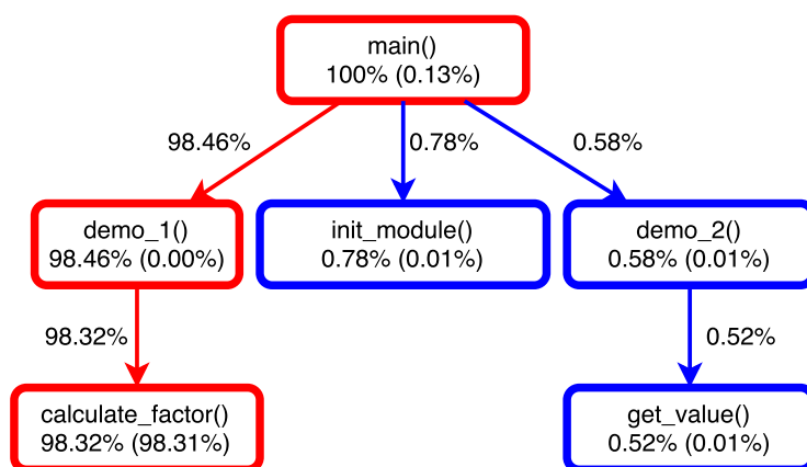
Obrázek 4.3: Graph view s vyznačenou kritickou cestou
