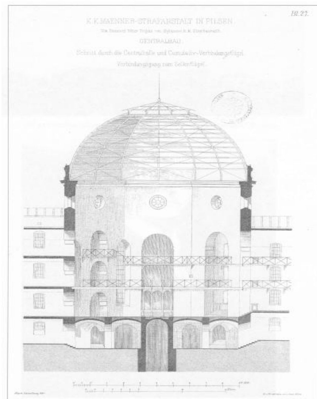
Průřez centrální budovy c. k. trestnice pro muže v Plzni, Allgemeine Bauzeitung (1881).
