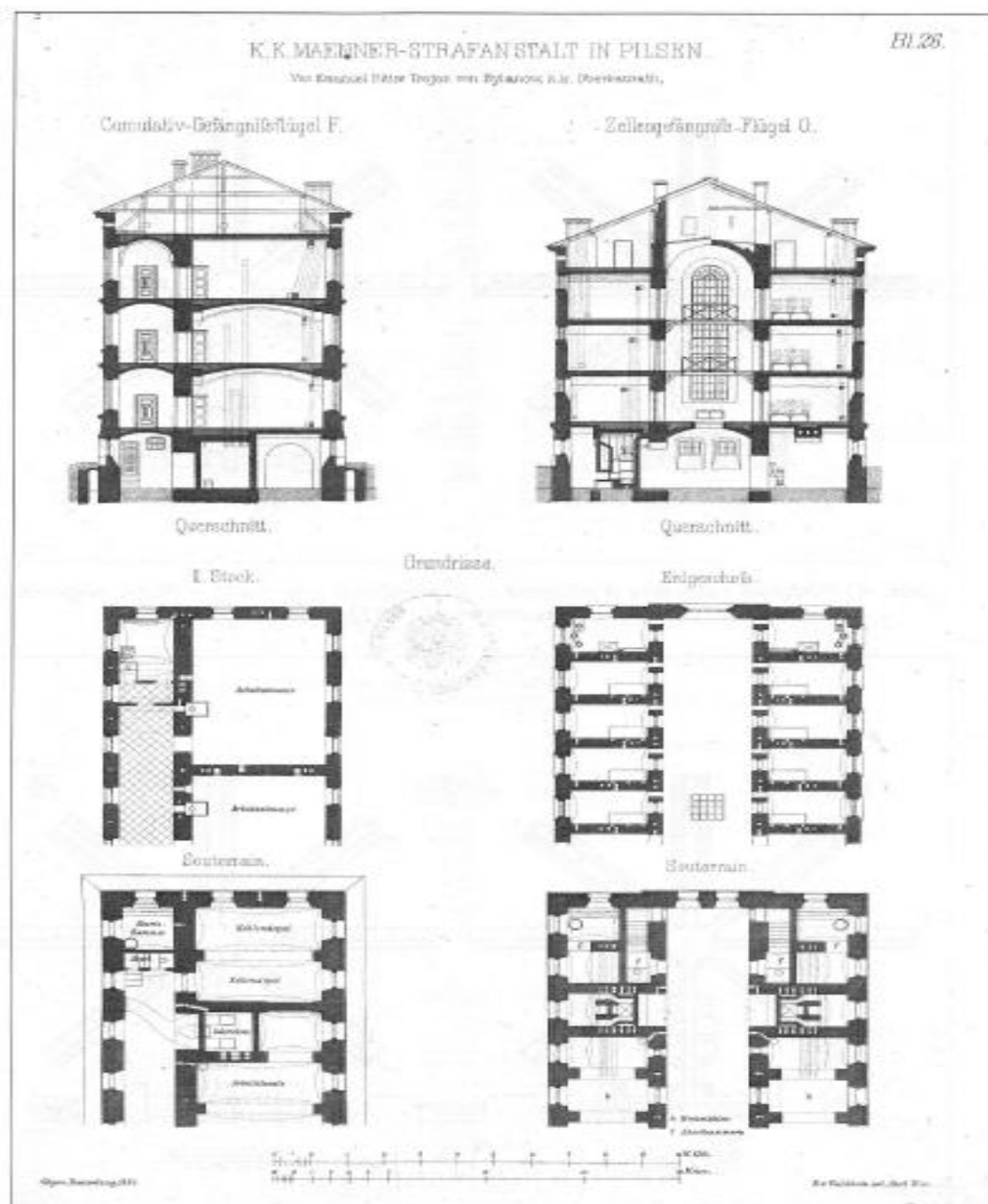
Průřez jednotlivými křídly c. k. trestnice pro muže v Plzni, Allgemeine Bauzeitung (1881).
