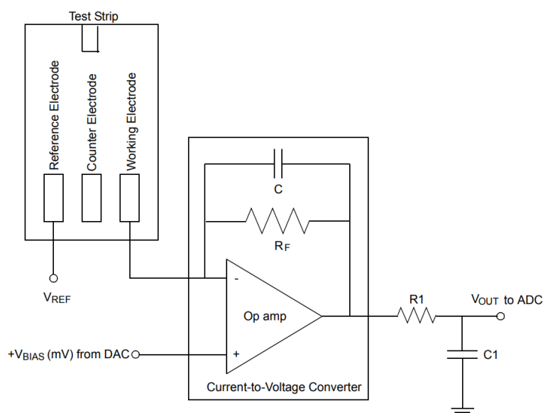
Obrázek 4.1: Schematické znázornění měřicí části přístroje, která převádí proud vzniklý na elektrodách na napětí, které lze převodníkem transformovat na číslo. Zde v aplikaci glukometru pro měření koncentrace glukózy v krvi. Obrázek převzat z [8]
