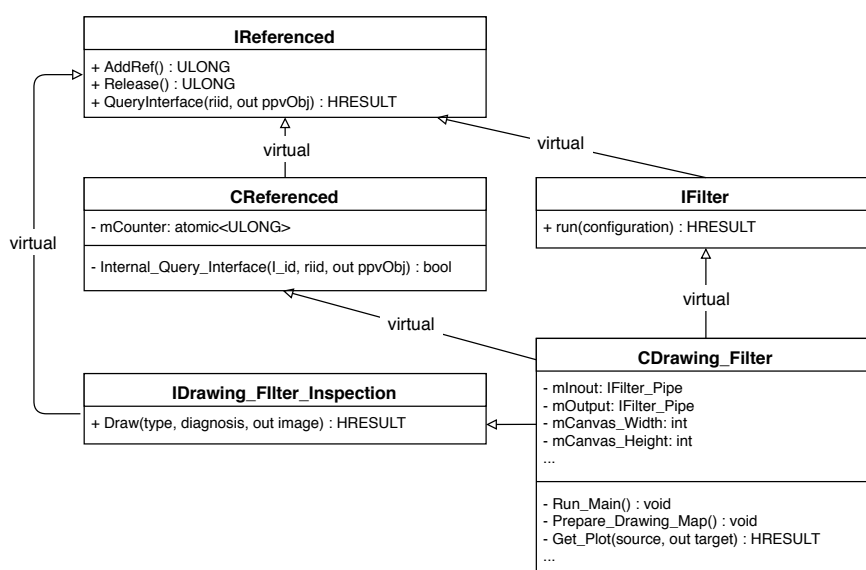
Obrázek A.6: UML diagram tříd pro rozhraní filtrů a příklad jedné implementace (jejíž atributy a metody byly výrazně zredukovány)
