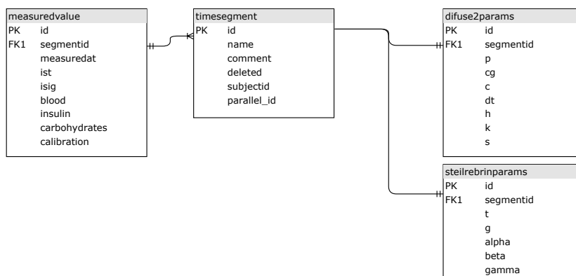
Obrázek 8.1: Schéma části databáze podstatné pro tuto práci
