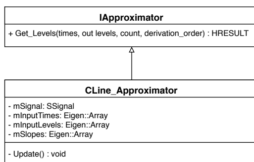
Obrázek A.5: UML diagram tříd pro rozhraní a implementaci aproximace a interpolace
