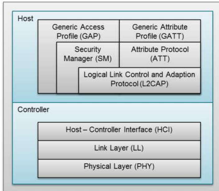
Obrázek 4.2: Bluetooth Low-Energy protokolový zásobník, dělení hostitelské a řídicí části. Obrázek převzat z [5]
