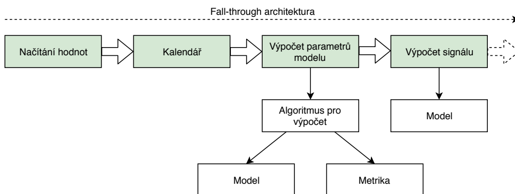
Obrázek 7.1: Příklad filtrů a vazeb na další moduly. Světle zeleně jsou označeny filtry ve fall-through architektuře
