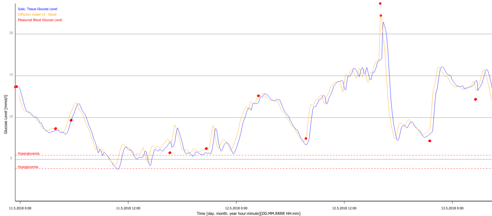
Obrázek 9.2: Graf vykreslený v aplikaci pro osobní počítač pro testovaný měřený segment; parametry byly spočítány ze všech dostupných hodnot segmentu algoritmem metadiferenciální evoluce s metrikou Crosswalk
