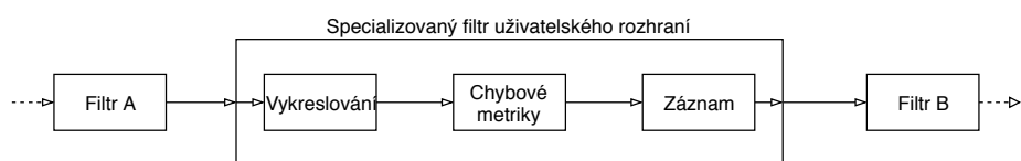
Obrázek 8.2: Schéma části filtrového řetězu, ve kterém figuruje i specializovaný filtr uživatelského rozhraní a jím obalené filtry
