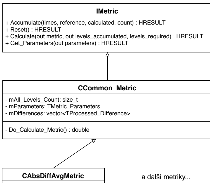
Obrázek A.7: UML diagram tříd pro rozhraní metrik, společného předka implementací a příklad jedné implementace
