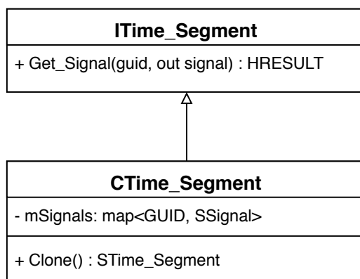
Obrázek A.3: UML diagram tříd pro rozhraní a implementaci časových segmentů
