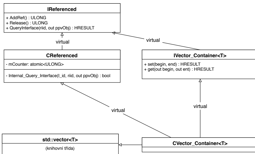
Obrázek A.1: UML diagram tříd pro rozhraní a implementaci meziknihovního čítání odkazů
