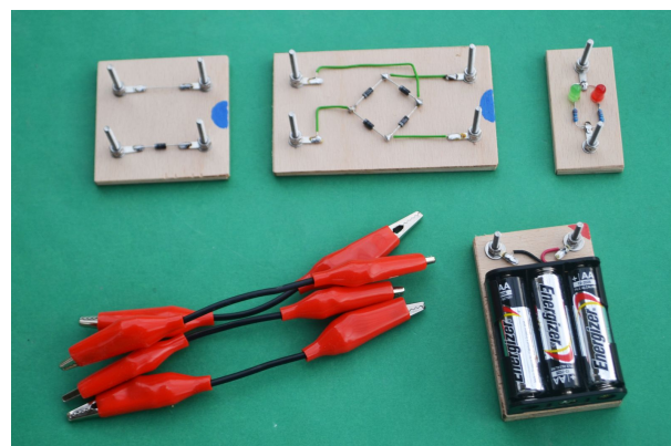
Obrázek 37: Žák. sada pro usměrnění
