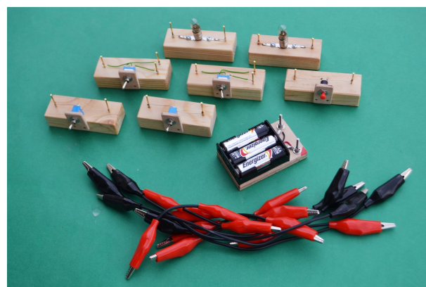
Obrázek 8: Žákovská sada el. obvodů
