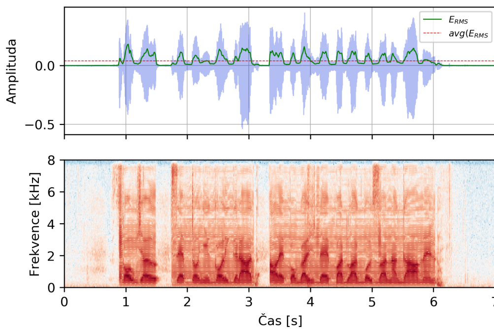
Obrázek 5.2: Průběh a spektrogram promluvy obsahující slovo „kosa“ s vyznačenou energií EL promluvy.
