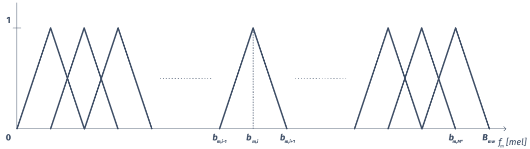
Obrázek 3.7: Rozložení banky trojúhelníkových filtrů v melovské frekvenční škále.
