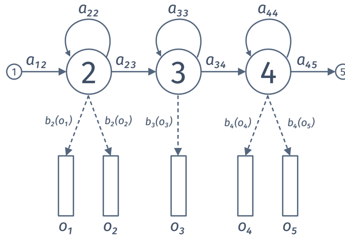
Obrázek 3.11: Příklad levo-právého Markovova modelu trifónu.
