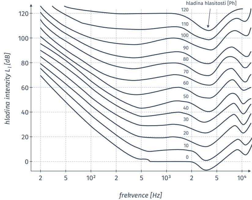
Obrázek 3.6: Křivky stejné hlasitosti. L_p = 20 \log(p/p_0) , p_0 = 2 \cdot 10^{-5} Pa .
