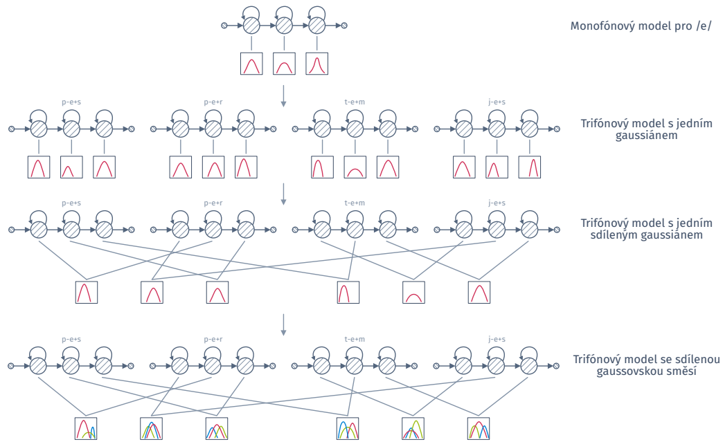
Obrázek 4.7: Princip trénování HMM-GMM modelu.
