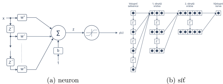
Obrázek 3.18: Neuron TDNN sítě a zjednodušené blokové schéma TDNN sítě [26].
