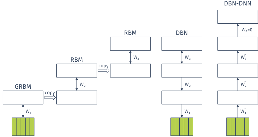
Obrázek 3.17: Princip předtrénování pomocí RBM s třemi vrstvami [22].
