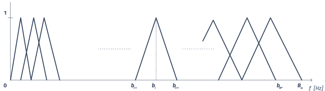
Obrázek 3.8: Rozložení banky trojúhelníkových filtrů ve frekvenční škále.
