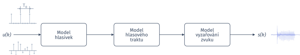
Obrázek 3.2: Blokové schéma modelu produkce řeči.
