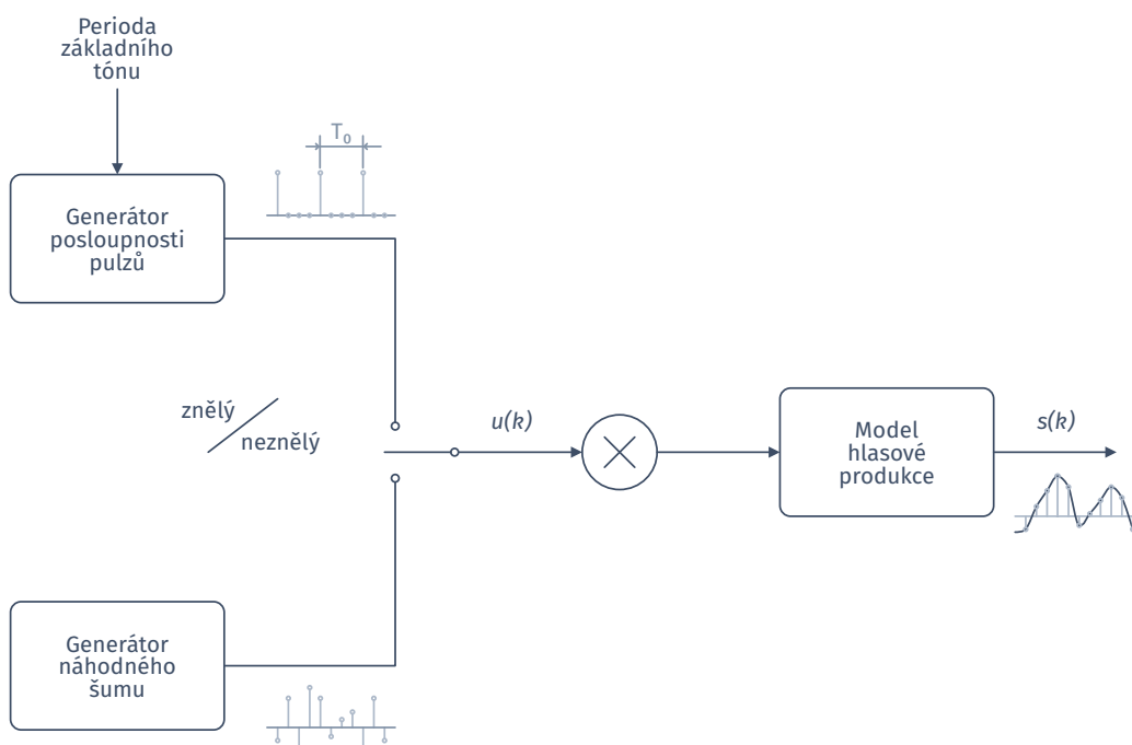
Obrázek 3.3: Blokové schéma upraveného modelu produkce řeči.
