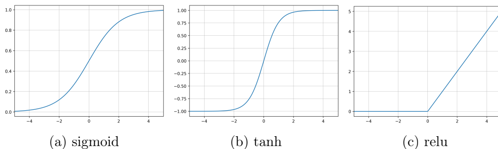
Obrázek 3.15: Příklady používaných aktivačních funkcí.
