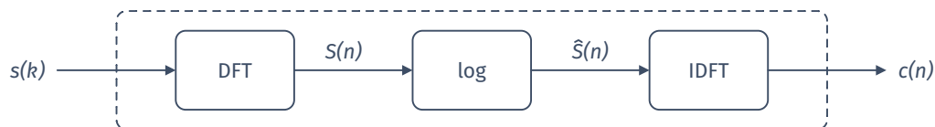
Obrázek 3.4: Blokové schéma principu výpočtu kepra.
