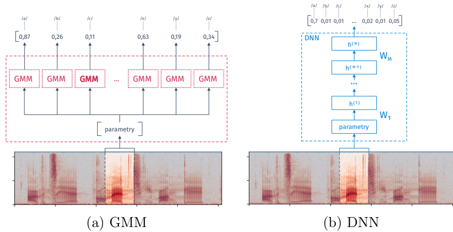
Obrázek 3.16: Principiální rozdíl ve funkci GMM a DNN systému.
