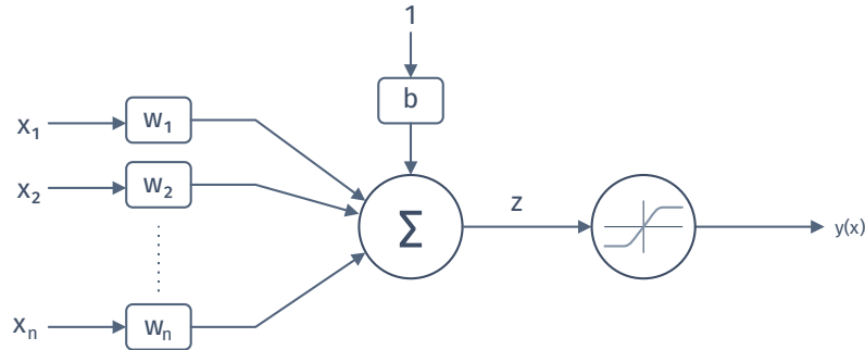
Obrázek 3.13: Schéma perceptronu.
