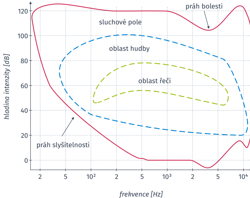
Obrázek 3.5: Charakteristické oblasti vnímání akustického signálu lidským sluchem. L_p = 20 \log(p/p_0) , p_0 = 2 \cdot 10^{-5} Pa .
