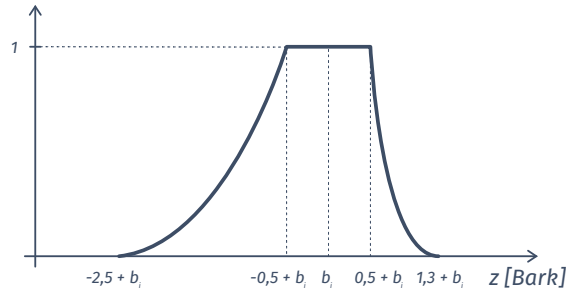
Obrázek 3.9: Ukázka filtru umístěného na Barkově frekvenční ose.
