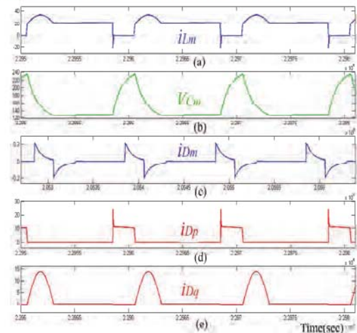
Figure 8 Simulated waveforms (a) i_{Lm} (b) V_{Cm} (c) i_{Dm} (d) i_{Dp} (e) i_{Dq}
