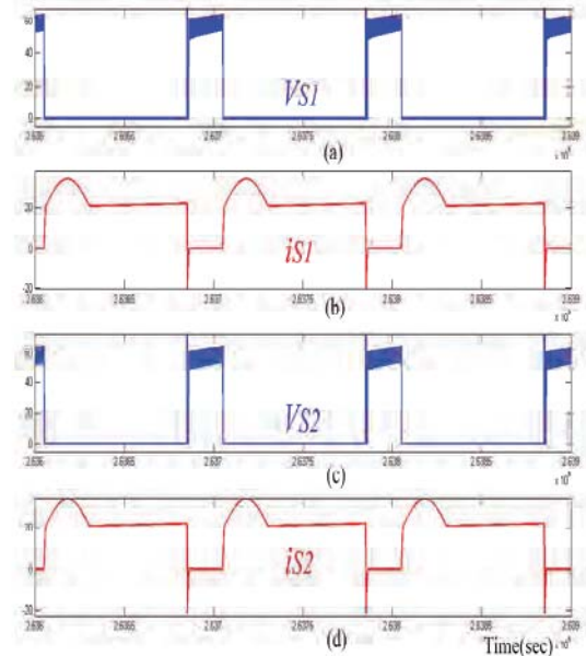
Figure 7 Simulated waveforms (a) V_{S1} (b) i_{S1} (c) V_{S2} (d) i_{S2}
