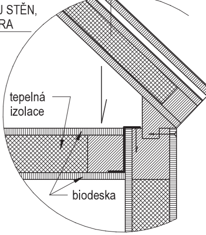
SKLADBA A SPOJ STĚN A PODLAHY
