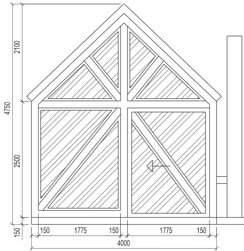
ČELNÍ POHLED
