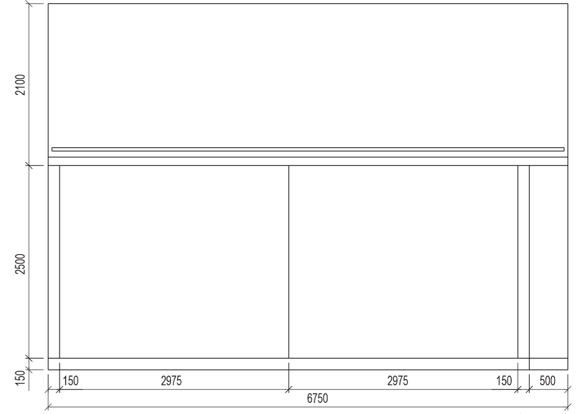
LEVÝ BOKORYSNÝ POHLED
