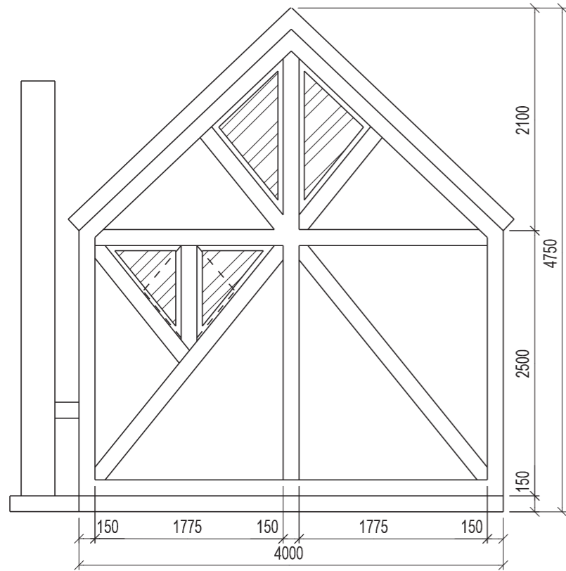
ZADNÍ POHLED
