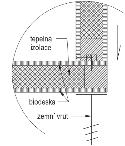
SKLADBA A SPOJ STĚN A PODLAHY
