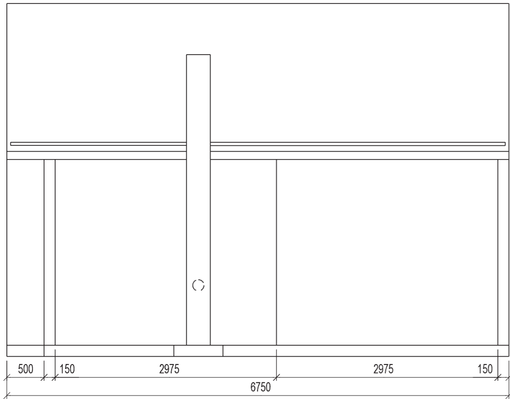
PRAVÝ BOKORYSNÝ POHLED
