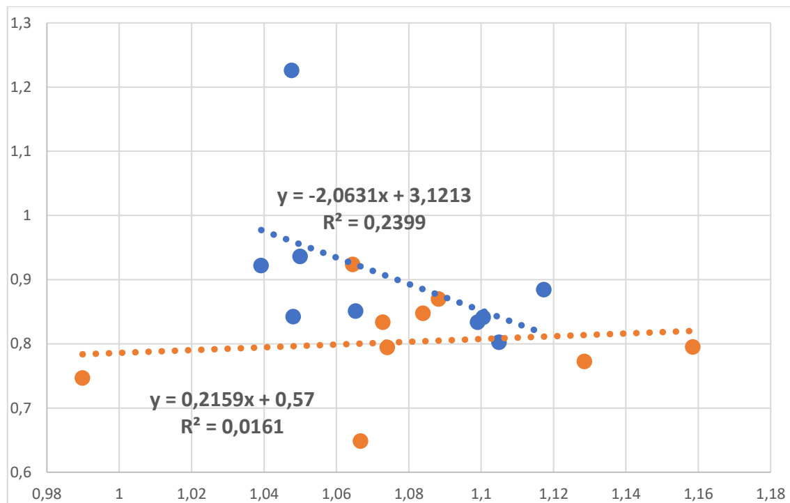
Obr. 25: Regresní analýza
