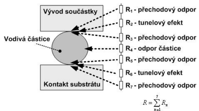
Obr. 2: Mechanizmy podílející se na vodivosti elektricky vodivého lepidla s anizotropní elektrickou vodivostí
