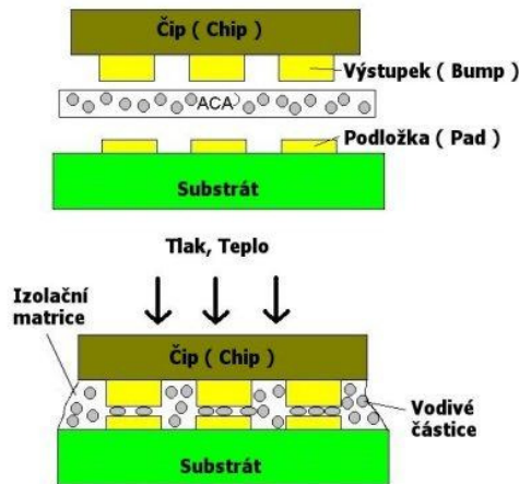
Obr. 1: Princip elektricky vodivého lepidla s anizotropní elektrickou vodivostí
