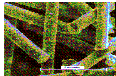
Obr. 5: Bazaltová vlákna pokrytá stříbrem
