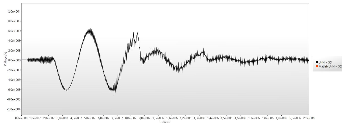
Obr. 12: Porovnání napětí pro N = 50 s Matlabem
