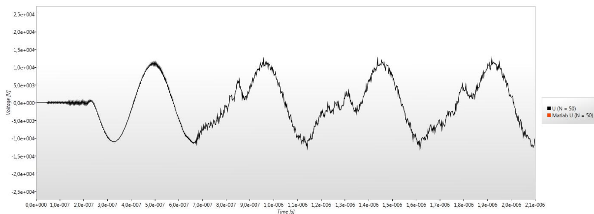
Obr. 24: Porovnání napětí pro N = 50 s Matlabem
