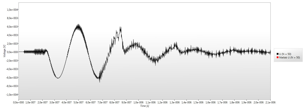
Obr. 18: Porovnání napětí pro N = 50 s Matlabem
