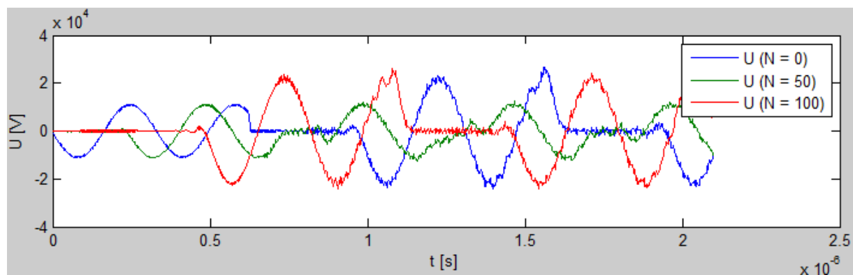
Obr. 19: Napětí v čase pro různé body vedení
