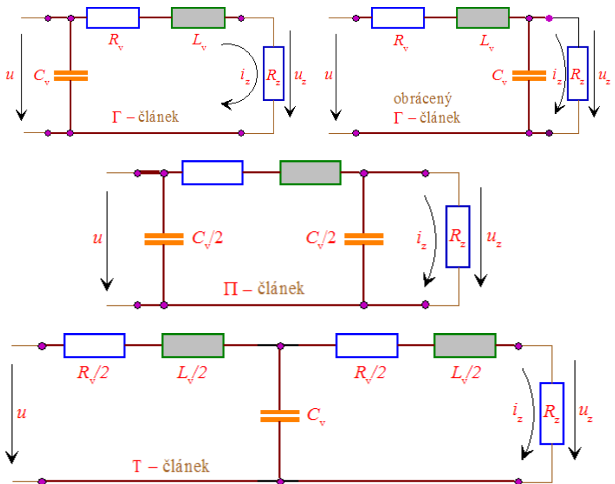
Obr. 1: Příklady náhradních obvodů [4]
