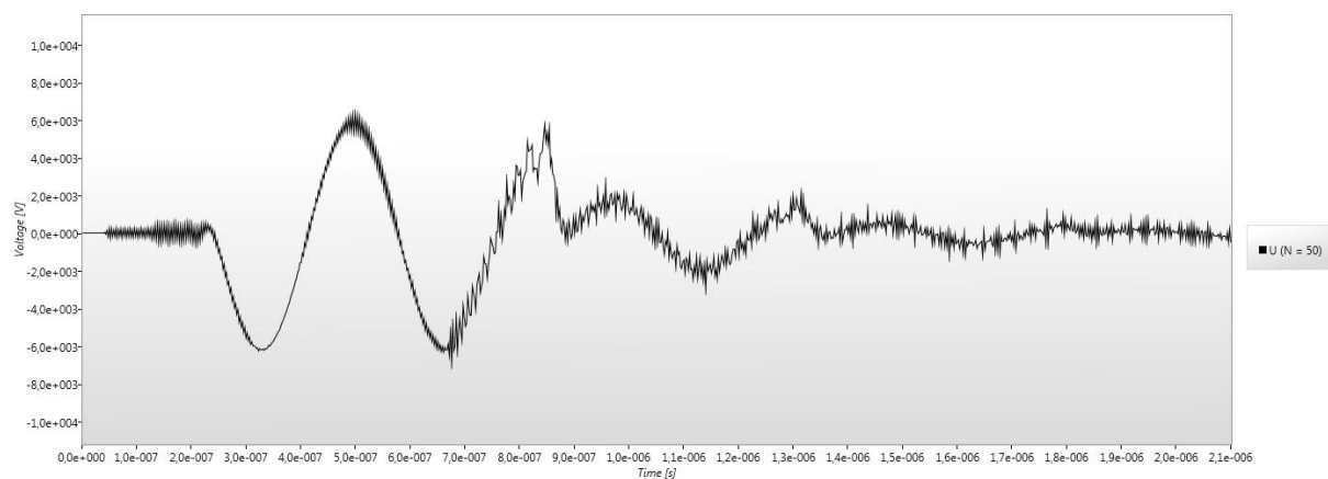
Obr. 16: Napětí v čase pro N = 50
