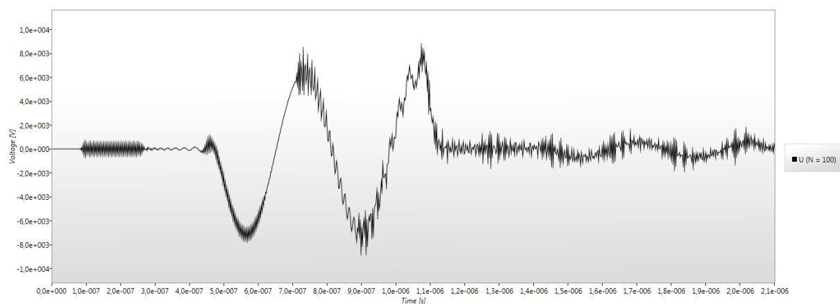
Obr. 17: Napětí v čase pro N = 100
