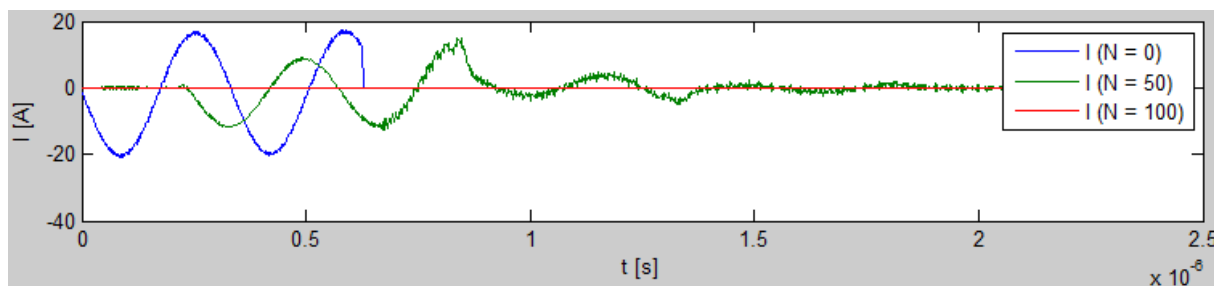
Obr. 14: Proud v čase pro různé body vedení
