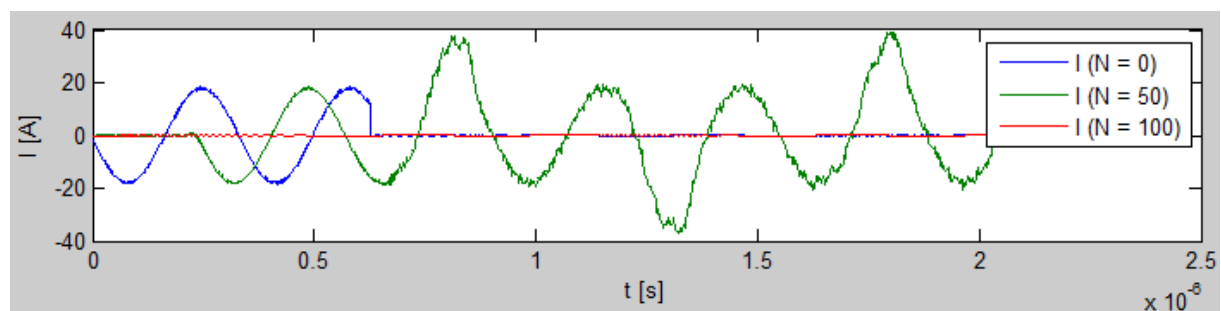
Obr. 20: Proud v čase pro různé body vedení
