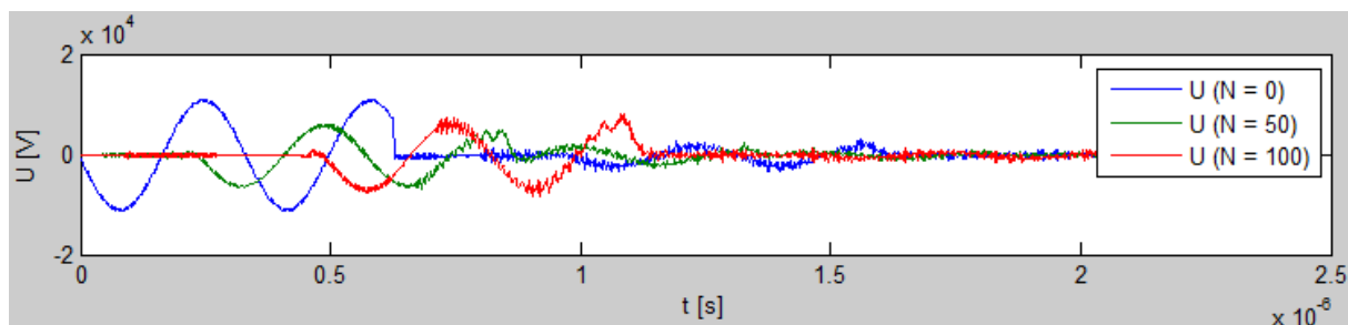
Obr. 13: Napětí v čase pro různé body vedení
