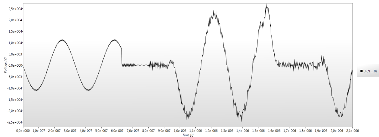
Obr. 21: Napětí v čase pro N = 0
