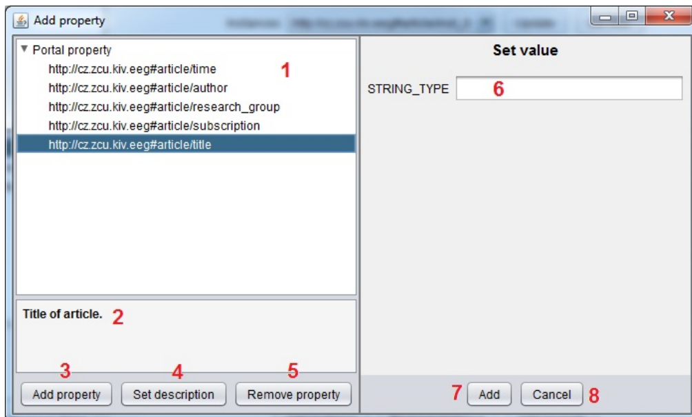
Obrázek A.7: Okno nastavení predikátů
