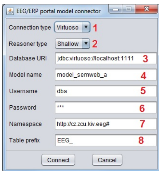
Obrázek A.2: Okno připojení testovací aplikace
