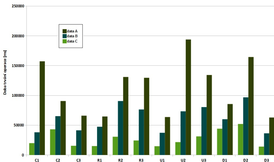
Obrázek 9.5: Doby trvání operací v závislosti na velikosti testovacích dat pro mělký reasoner nad databází Oracle
