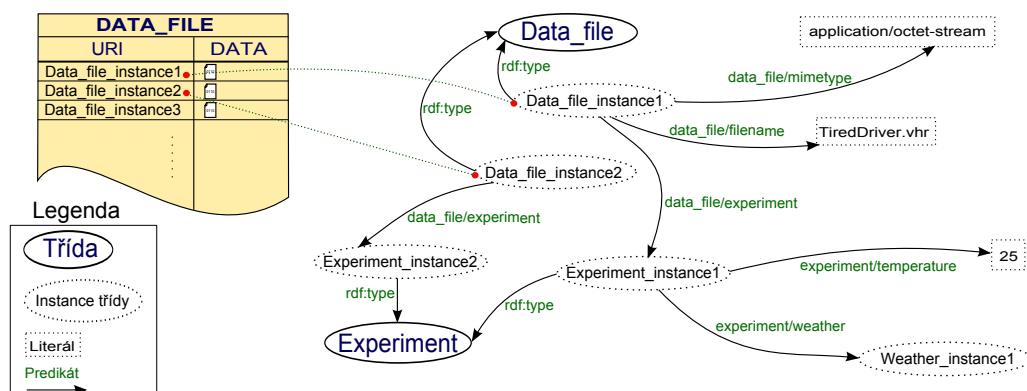
Obrázek 7.4: Znázornění částí výsledného modelu
