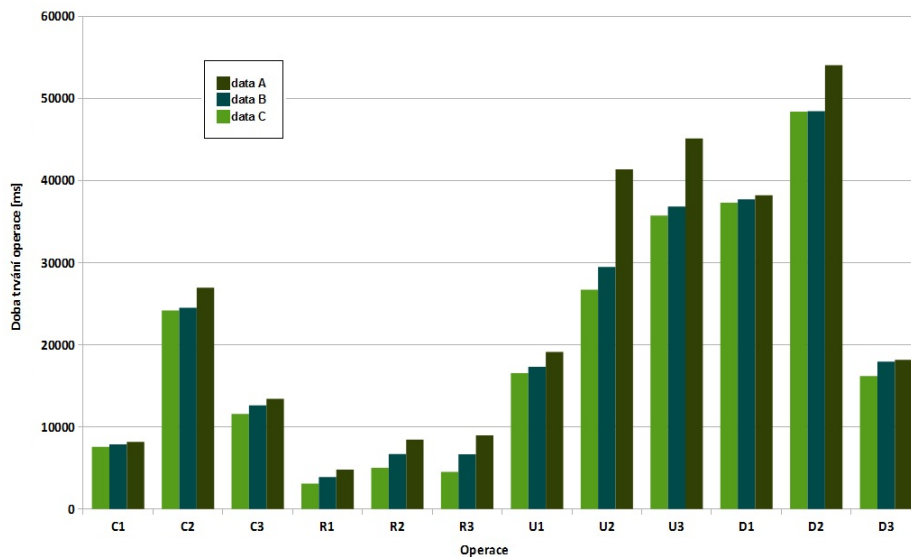
Obrázek 9.4: Doby trvání operací v závislosti na velikosti testovacích dat pro hluboký reasoner nad databází Virtuoso
