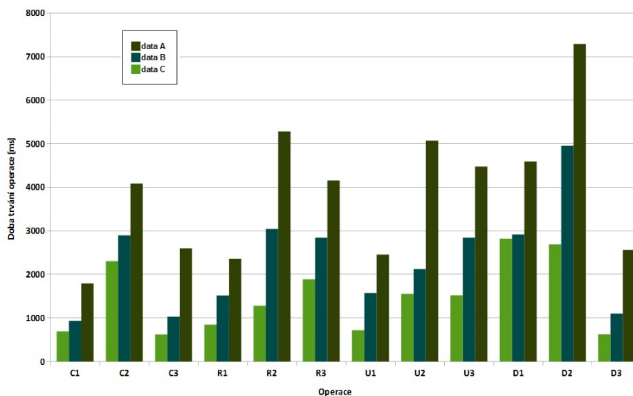
Obrázek 9.3: Doby trvání operací v závislosti na velikosti testovacích dat pro mělký reasoner nad databází Virtuoso
