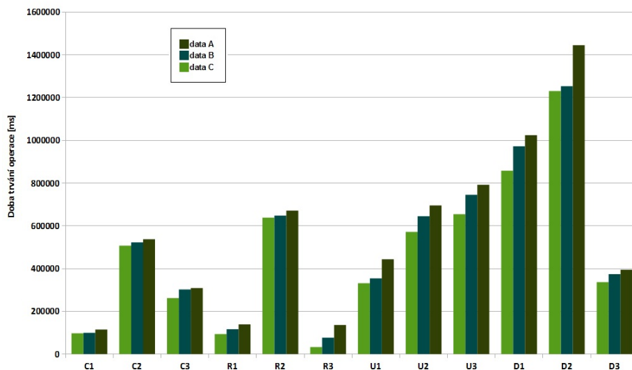
Obrázek 9.6: Doby trvání operací v závislosti na velikosti testovacích dat pro hluboký reasoner nad databází Oracle
