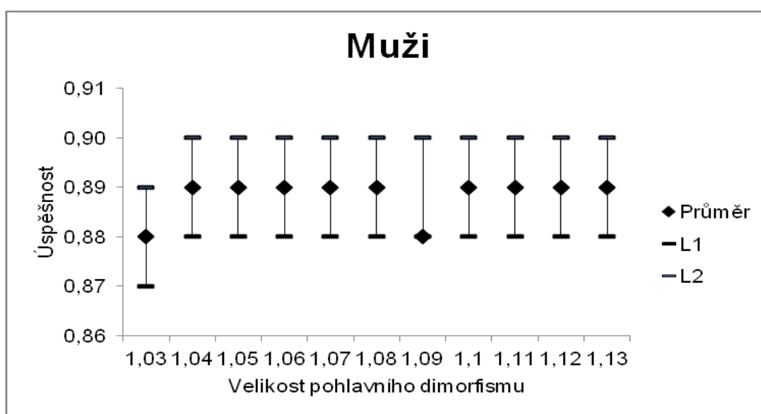
Graf č. 13. Závislost úspěšnosti metody na míře pohlavního dimorfismu u mužů při změně směrodatné odchylky rozměrů žen
