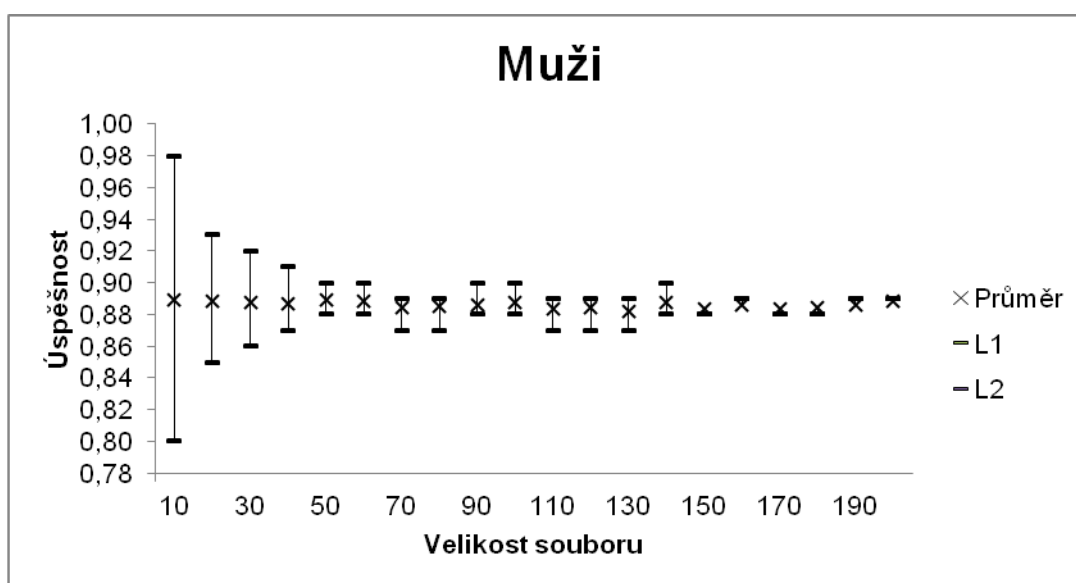
Graf č. 4. Závislost velikosti souboru na úspěšnosti při použití rozměru obvod kloubní hlavice pažní kosti pro muže
