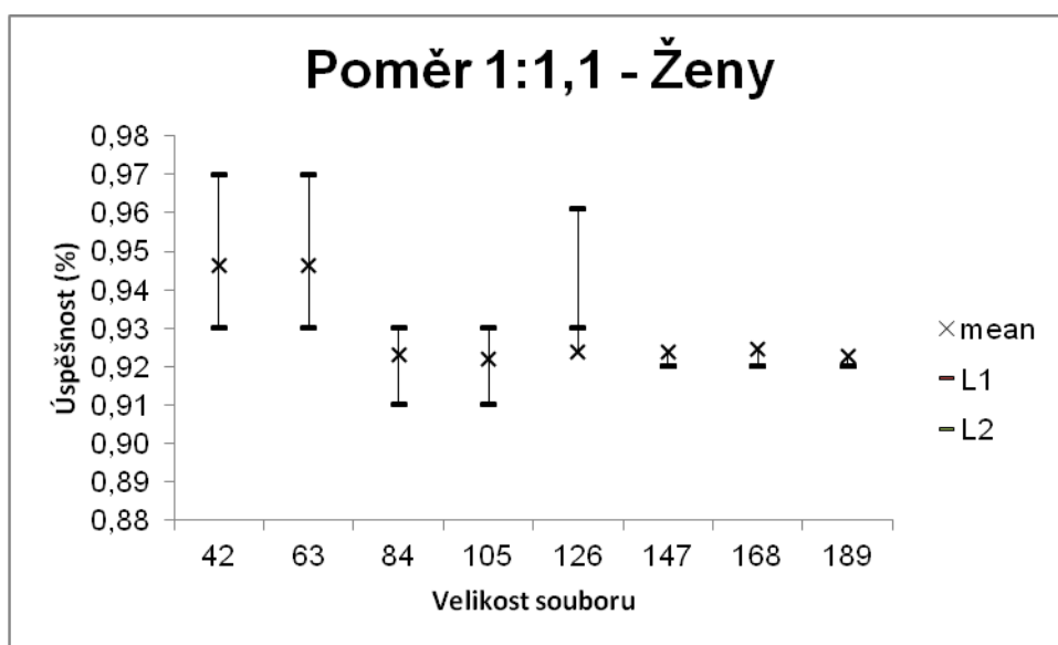
Graf č. 9 Závislost úspěšnosti metody na velikosti souboru při poměru mužů a žen 1:1,1
