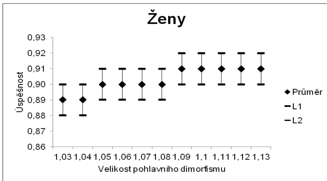
Graf č. 12. Závislost úspěšnosti metody na míře pohlavního dimorfismu u žen při změně směrodatné odchylky
