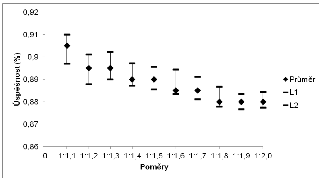
Graf č. 7. Závislost úspěšnosti metody na poměru pohlaví
