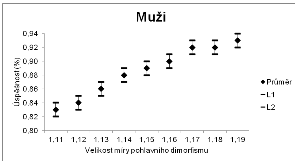
Graf č. 10. Závislost úspěšnosti metody na míře pohlavního dimorfismu u mužů při změně průměrů
