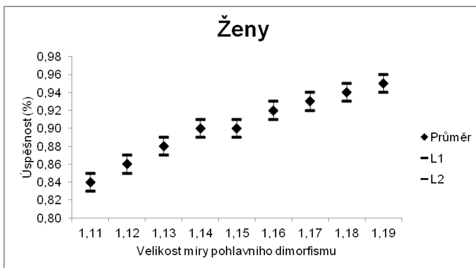
Graf č. 11. Závislost úspěšnosti metody na míře pohlavního dimorfismu u žen při změně průměrů
