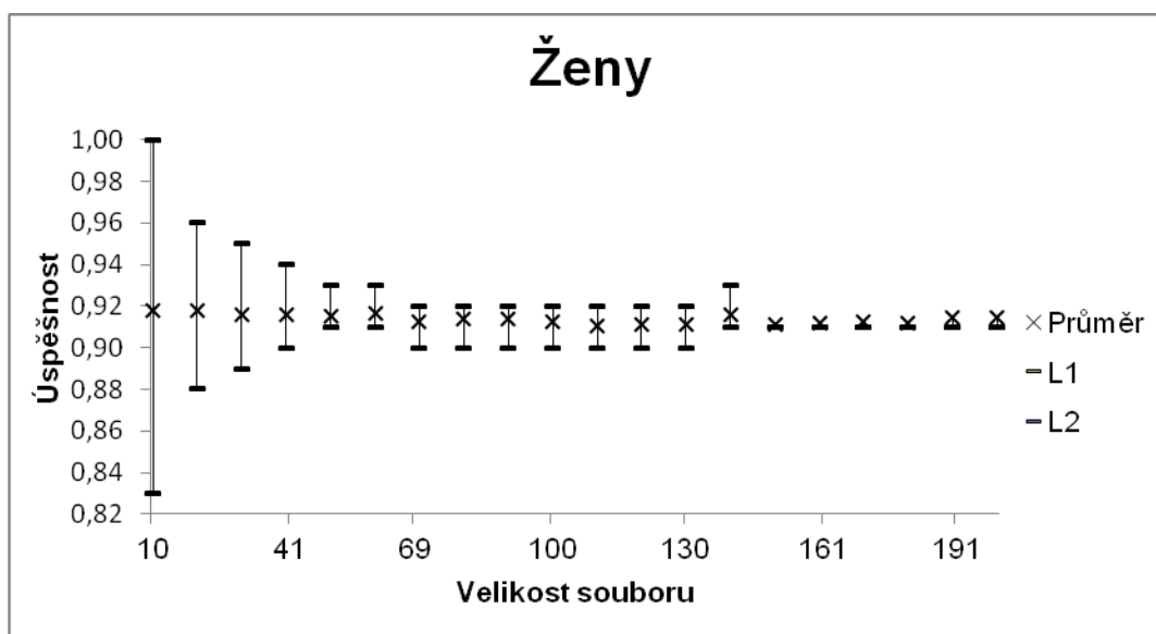
Graf č. 5. Závislost velikosti souboru na úspěšnosti při použití rozměru obvod kloubní hlavice pažní kosti pro ženy
