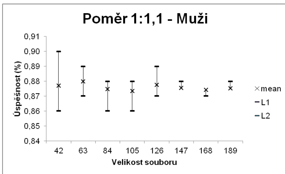
Graf č. 8. Závislost úspěšnosti metody na velikosti souboru při poměru mužů a žen 1:1,1
